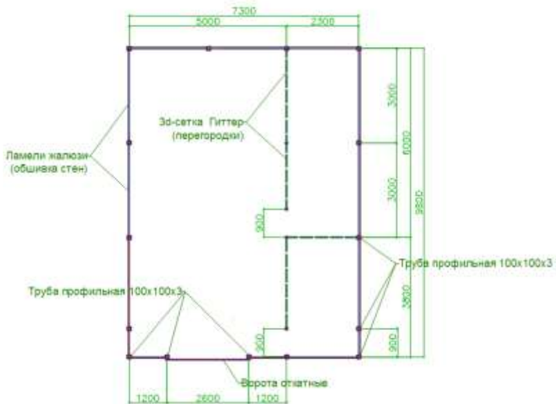
План контейнерной площадки ТБО №1
